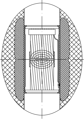
Рис.3 Сварное соединение (Опционально)
