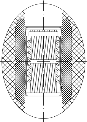
Рис.1 Опрессованное соединение (Стандартное исполнение)
