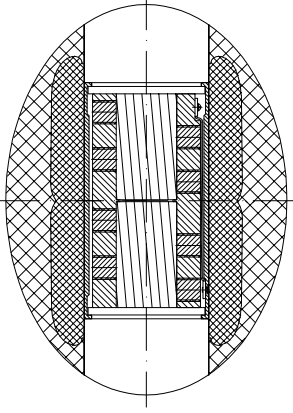
Рис.2 Винтовое соединение (Опционально)
