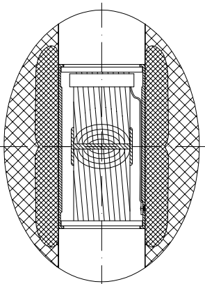
Рис.3 Сварное соединение (Опционально)
