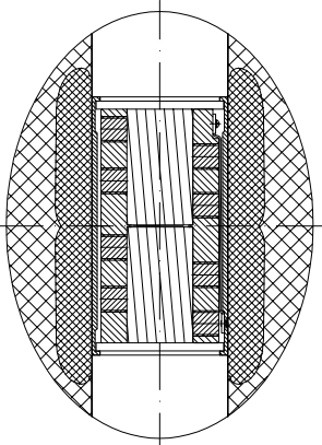
Рис.2 Винтовое соединение (Опционально)
