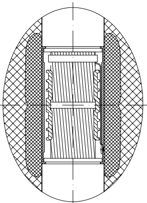
Рис.1 Опрессованное соединение (Стандартное исполнение)
