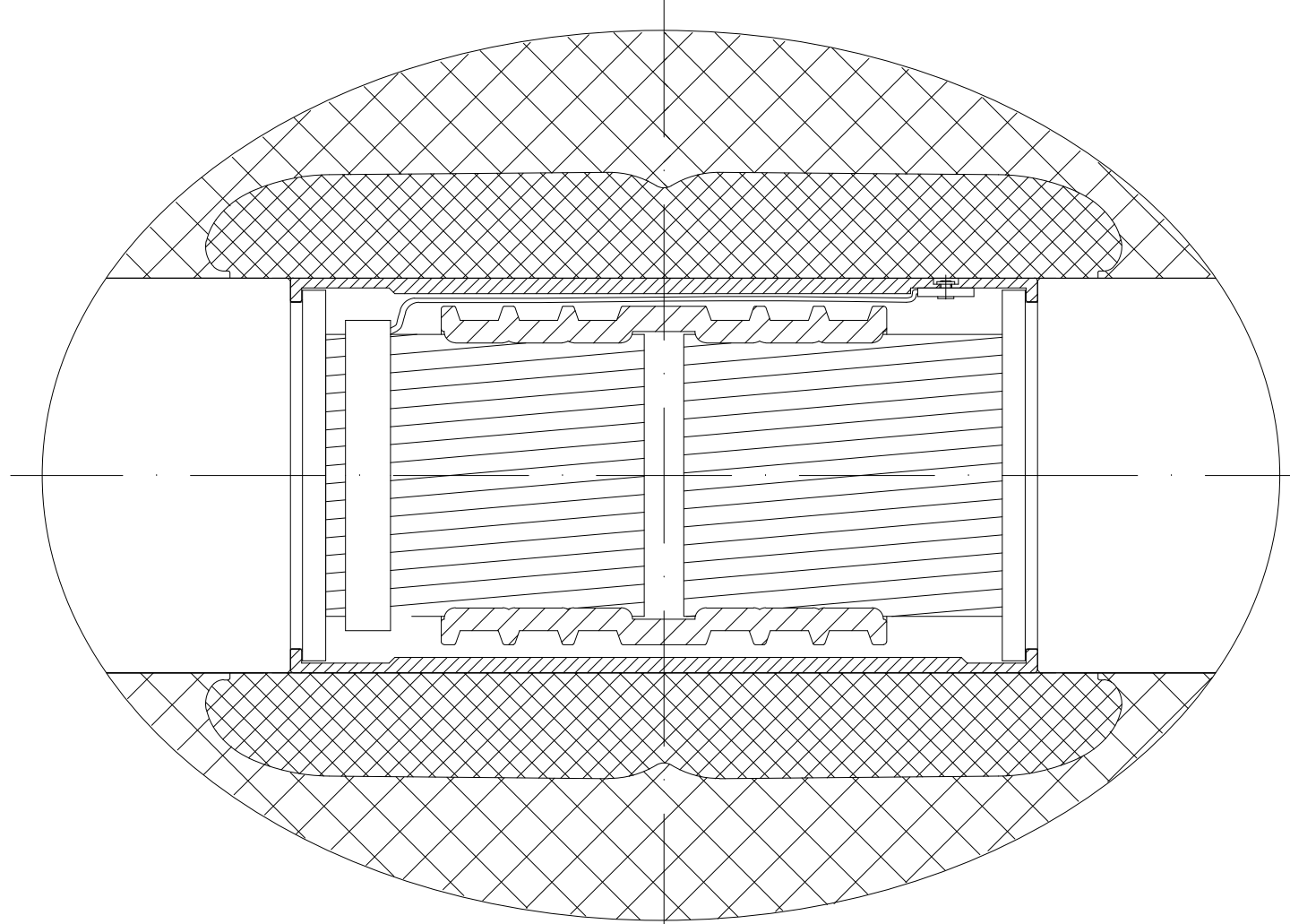
Рис.1 Опрессуемое соединение (Стандартное исполнение)
