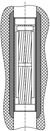
Рис.1 Опрессованное соединение (Стандартное исполнение)
