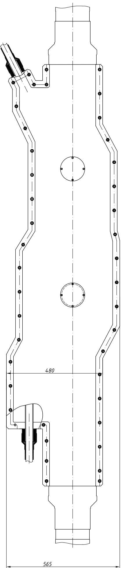
Рис.1 Опрессованное соединение (Стандартное исполнение)
