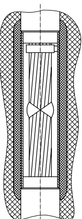
Рис.3 Сварное соединение (Опционально)
